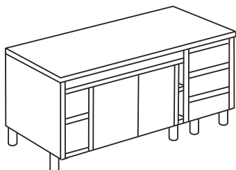
Zatvoreni radni stolovi sa kliznim vratima i fijokama
